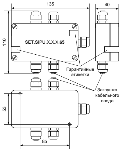
Рисунок А.2 – Внешний вид, габаритные и установочные размеры счётчика SET.SIPU.X.X.X.65
