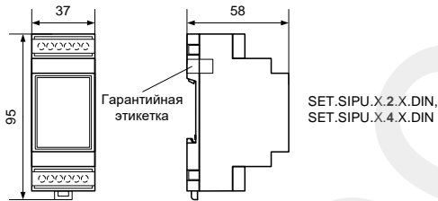
Рисунок А.3 – Внешний вид, габаритные и установочные размеры счётчиков SET.SIPU.X.2.X.DIN, SET.SIPU.X.4.X.DIN
