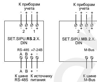
Рисунок А.7 – Схема подключения приборов учета ресурсов к счётчику SET.SIPU.X.2.X.DIN
