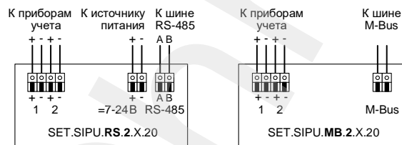
Рисунок А.5 – Схема подключения приборов учета ресурсов к счётчику SET.SIPU.X.2.X.20
