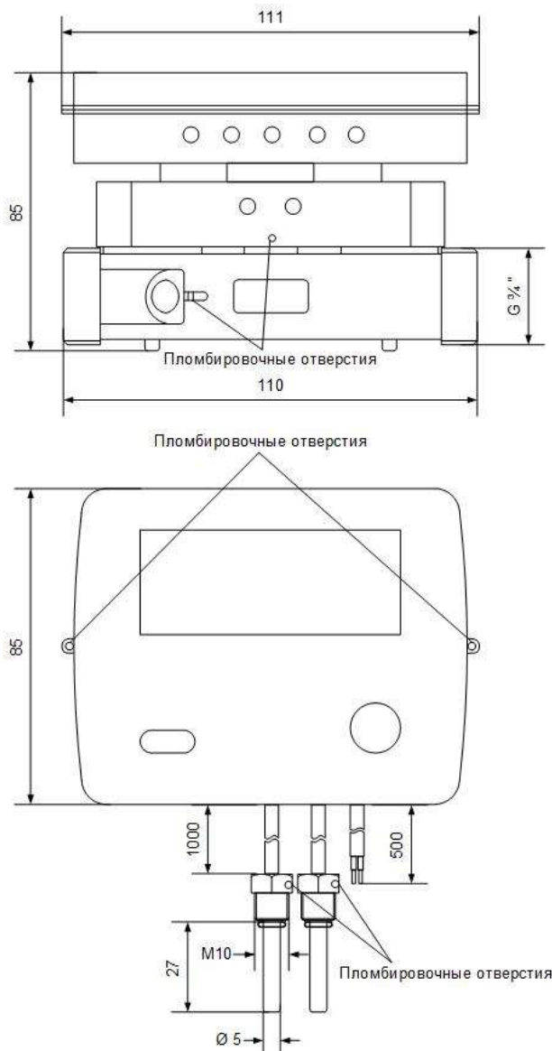
Рисунок 1. Теплосчётчик «ТСУ-15.хх»
