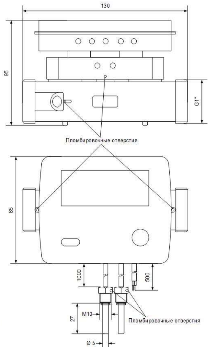
Рисунок 2. Теплосчётчик «ТСУ-20.хх»
