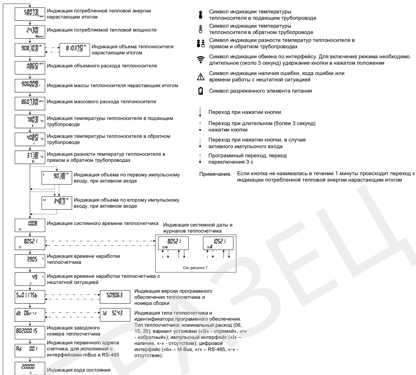
Рисунок 1. Последовательность переключения параметров на индикаторе теплосчетчика
