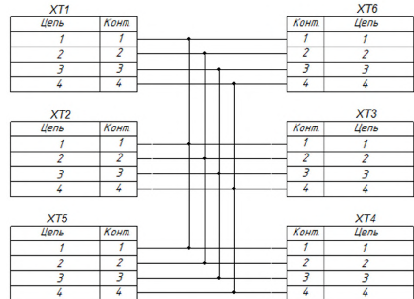
Разветвитель СЭТ.469333.091-06 Рис.7
