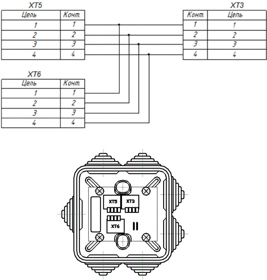
Разветвитель СЭТ.469333.091-08 Рис.9
