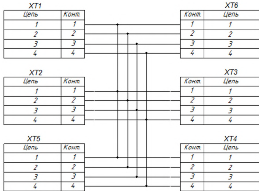
Разветвитель СЭТ.469333.091-03 Рис.4
