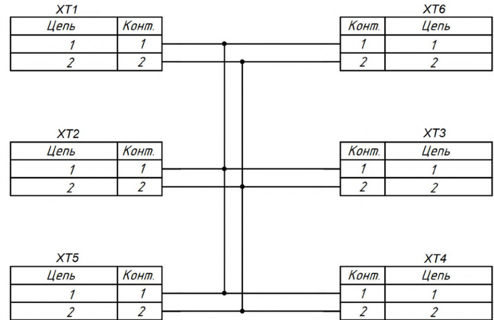
Разветвитель СЭТ.469333.091-04 Рис.5
