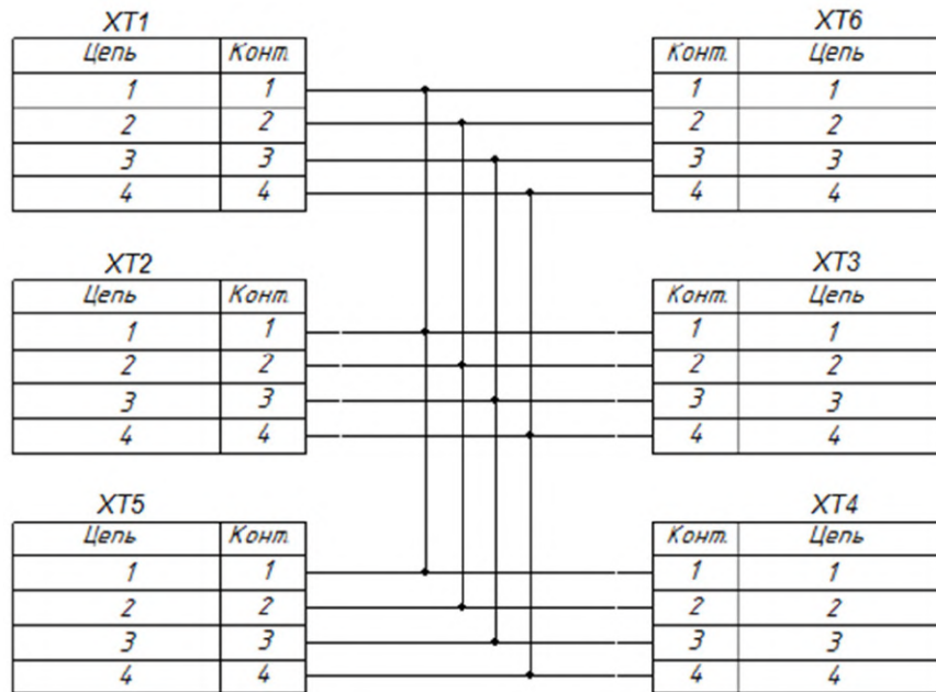
Разветвитель СЭТ.469333.091-01 Рис.2
