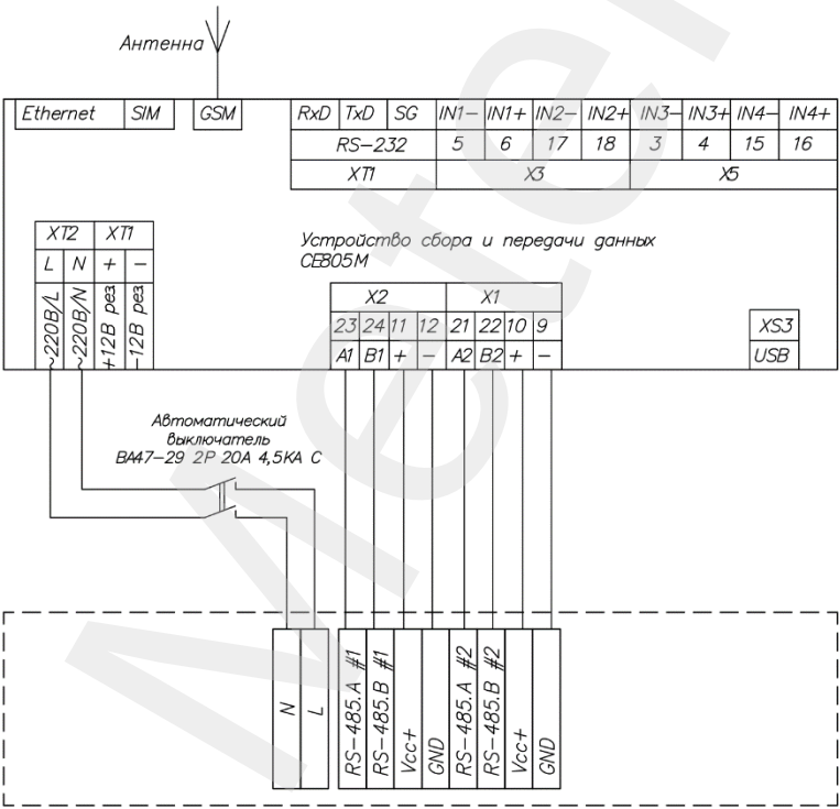
Рисунок 3 – Структурная схема щита автоматизации ЩА.240-02
