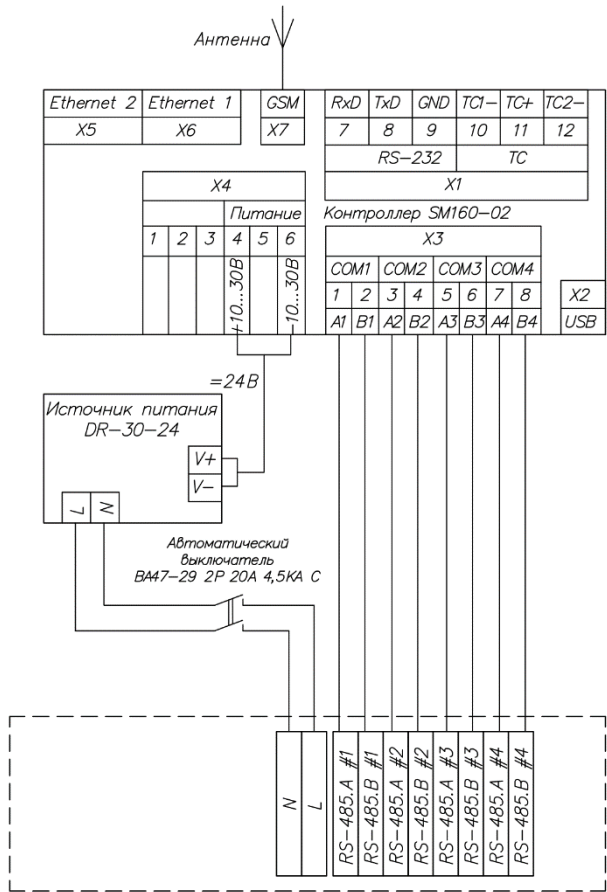
Рисунок 1 – Структурная схема щита автоматизации ЩА.240-00
