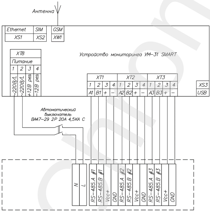
Рисунок 2 – Структурная схема щита автоматизации ЩА.240-01
