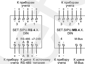
Рисунок А.8 – Схема подключения приборов учета ресурсов к счётчику SET.SIPU.X.4.X.DIN
